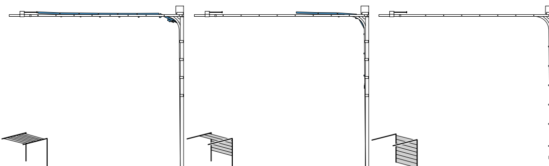
Verlauf Torblatt in verschiedenen Öffnungsstadien
