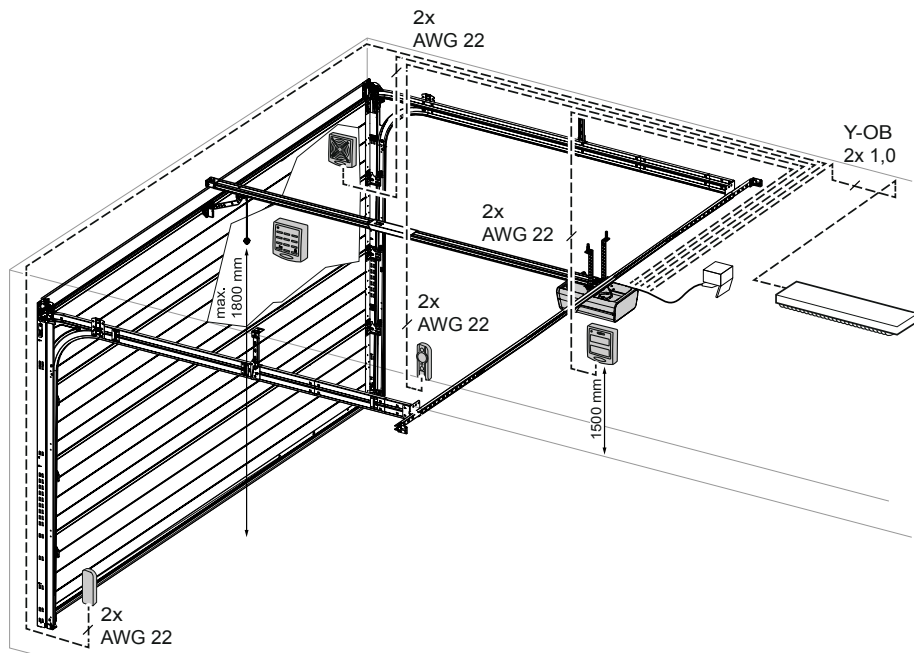
Abb. 3: Beispielinstallation Zubehör
