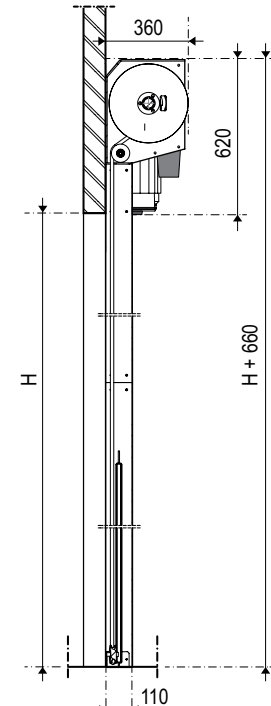
Schnitt 3-3
