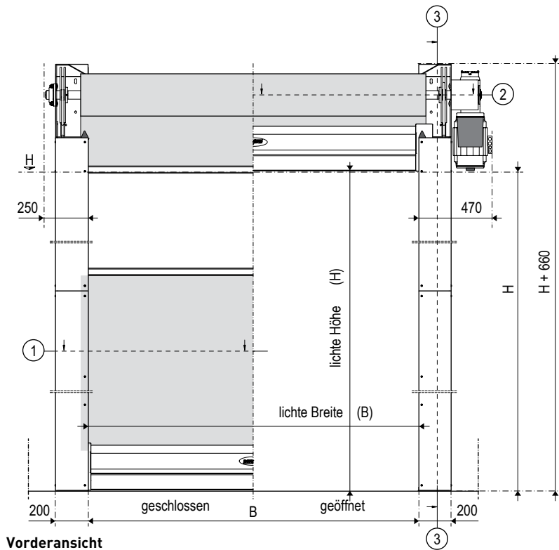
Vorderansicht
