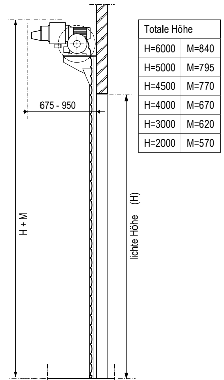
Vertikalschnitt
