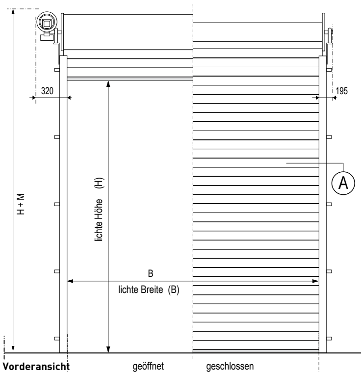
Vorderansicht
