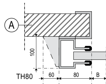
Vertikalschnitt
