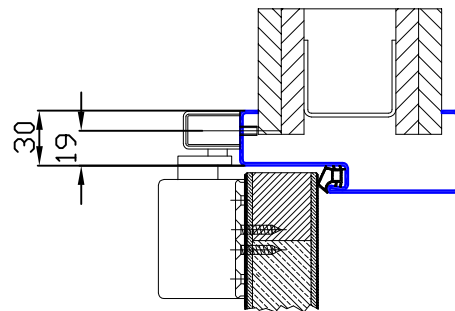
Standardausführung Mit Spiegelverbreiterung auf der Falzseite
