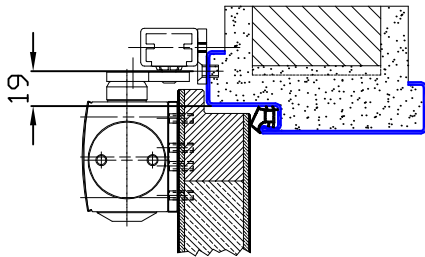
Standardausführung Vorgefertigt für bauseitige Scharnierplatte
