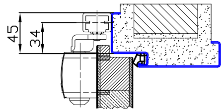
Sonderausführung Mit Spiegelverbreiterung auf der Falzseite
