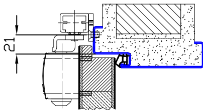
Standardausführung Vorgerichtet für bauseitige Scharnierplatte
