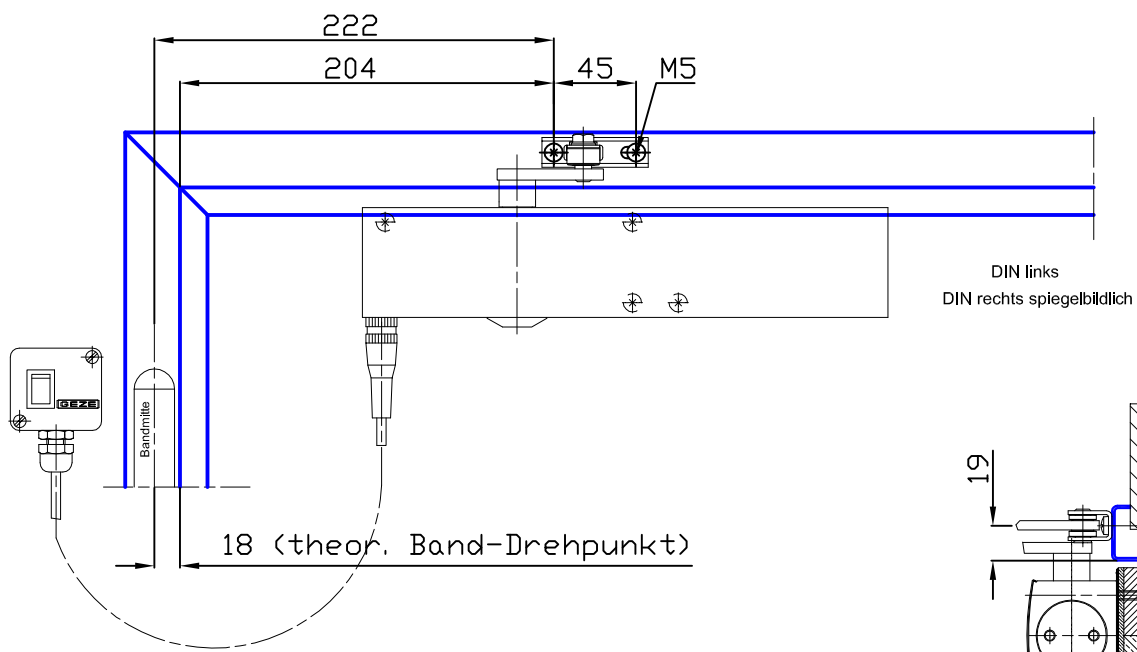
Standardausführung
