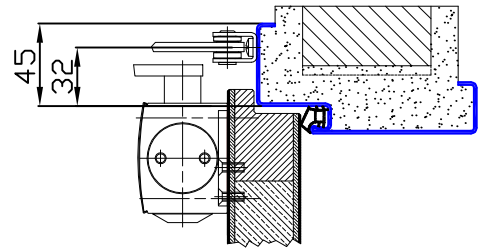
Sonderausführung Mit Spiegelverbreiterung auf der Falzseite
