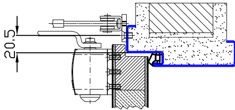
Standardausführung Vorgerichtet für bauseitige Scharnierplatte
