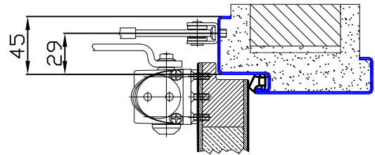
Sonderausführung Mit Spiegelverbreiterung auf der Falzseite
