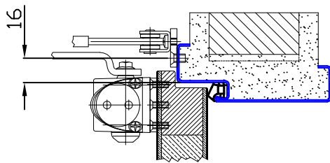
Standardausführung Vorgerichtet für bauseitige Scharnierplatte
