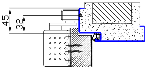
Standardausführung bei gefälzter Ausführung Mit Spiegelverbreiterung auf der Falzseite
