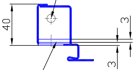
Anschweißblase 30 x 15 x 3
