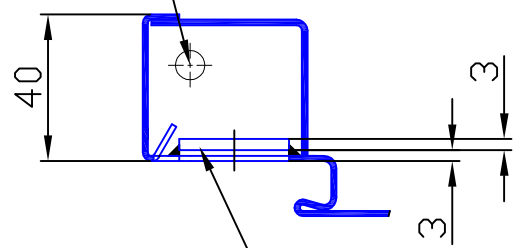
Anschweißblase 30 x 15 x 3
