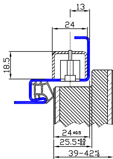
Zarge für gefälztes Türblatt
