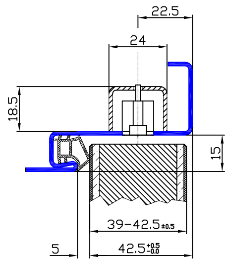
Zarge für ungefälztes Türblatt
