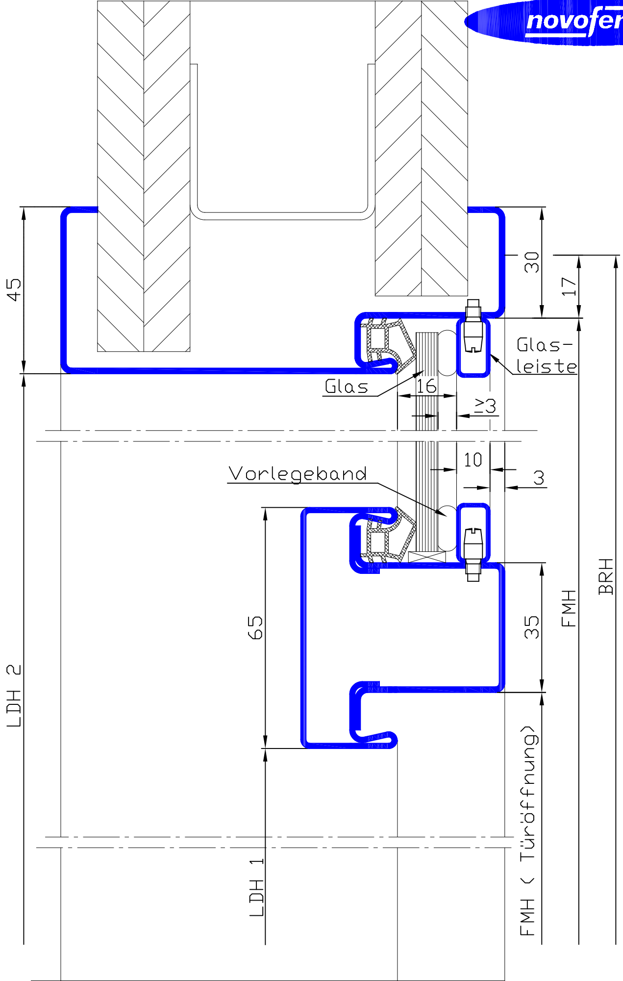
Verglasung und Vorlegeband bauseits
