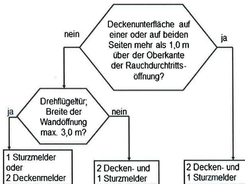
Bild 3: Entscheidungsdiagramm
