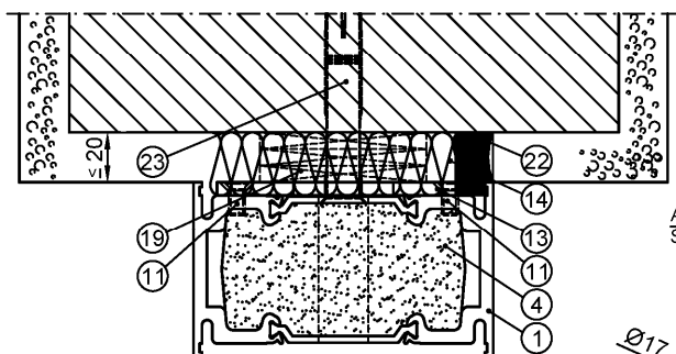
Dargestellt Durchsteckmontage, wahlweise Anschweißmontage
