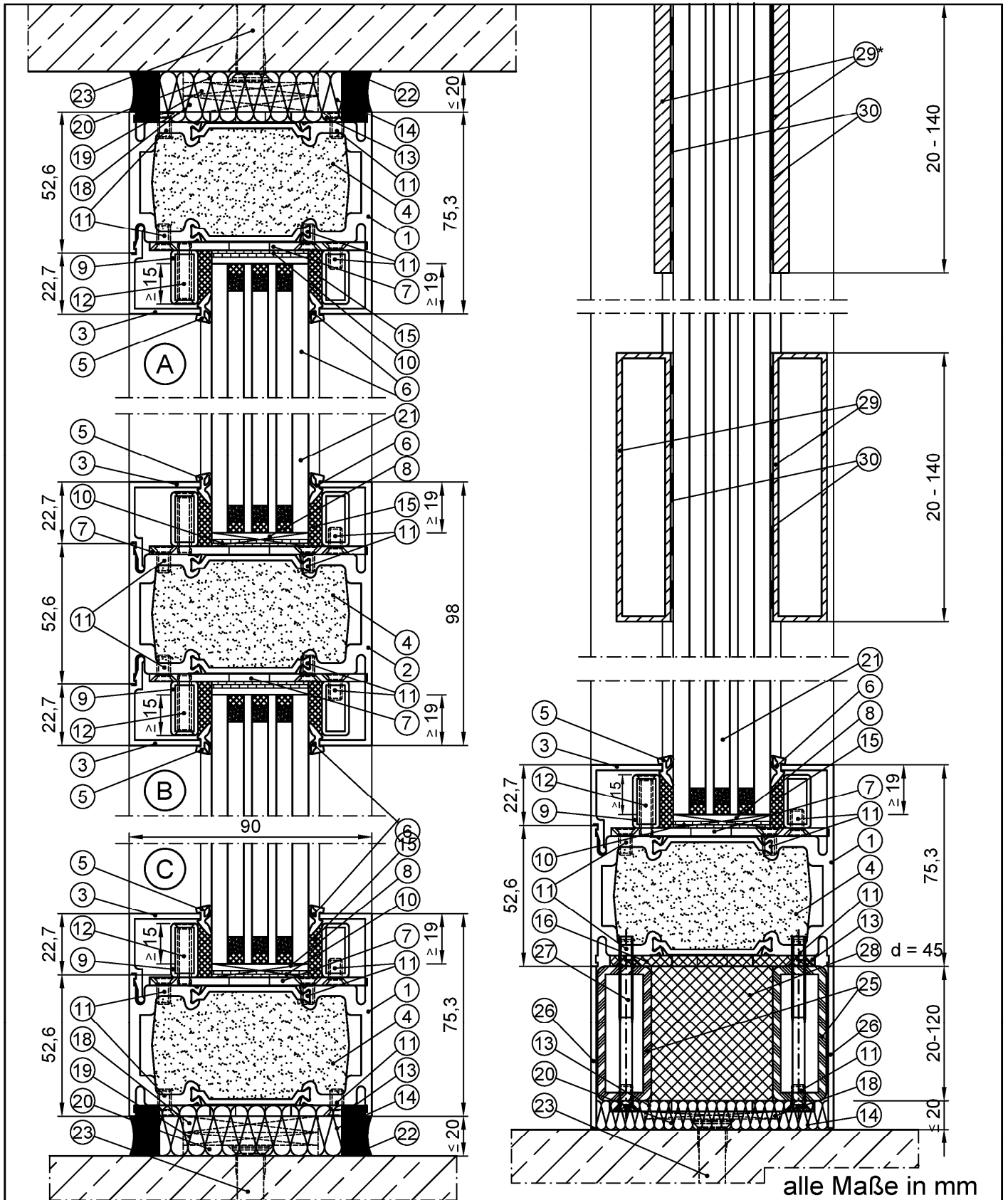
Bauart zum Errichten der Brandschutzverglasung "System NovoFire " der Feuerwiderstandsklasse F 90 nach DIN 4102-13
