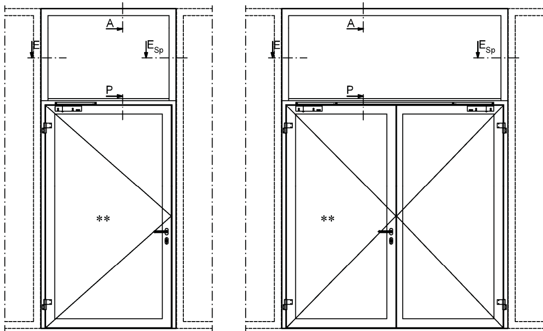
wahlweise Anschluss von Feuerschutzabschlüssen
