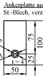
Dargestellt Anschweißmontage
