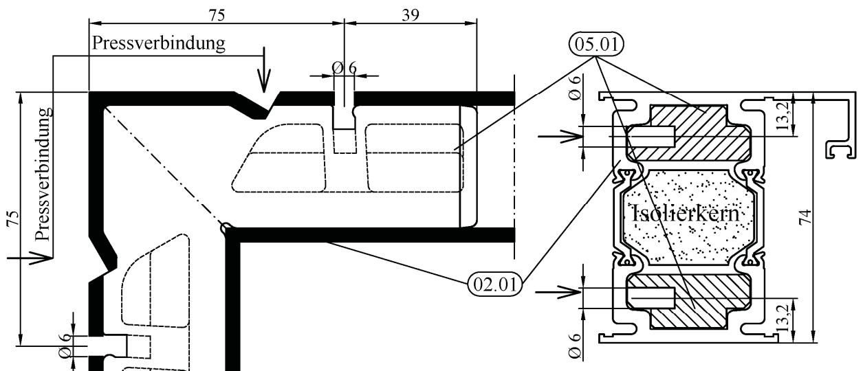
Eckwinkel mit Metallkleber der Firma Weiss - Chemie + Technik GmbH Verkleben und Verpressen oder wahlweise Verstiften der Verbindung anstelle verpressen.
