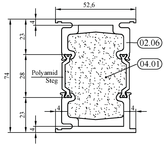
Glasleiste aussen, anschraubbar Profil.-Nr. 27952
