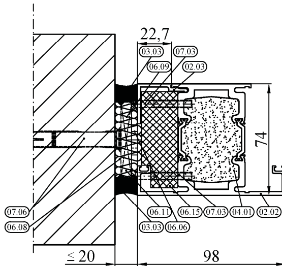
Dargestellt Anschweißmontage
