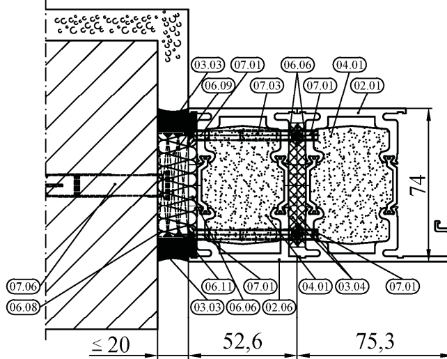
Dargestellt Anschweißmontage
