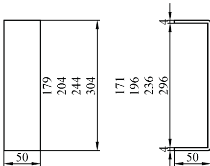
Dargestellt Durchsteckmontage, wahlweise Anschweißmontage
