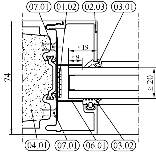
Scheibe "POLFLAM EI 30"
