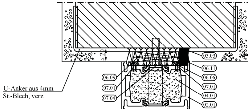
Dargestellt Durchsteckmontage, wahlweise Anschweißmontage
