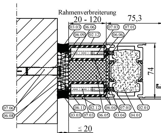
Dargestellt Anschweißmontage
