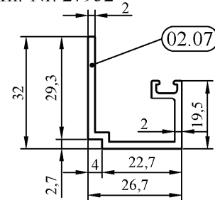
Glasleiste aussen, anschraubbar Profil.-Nr. 27952
