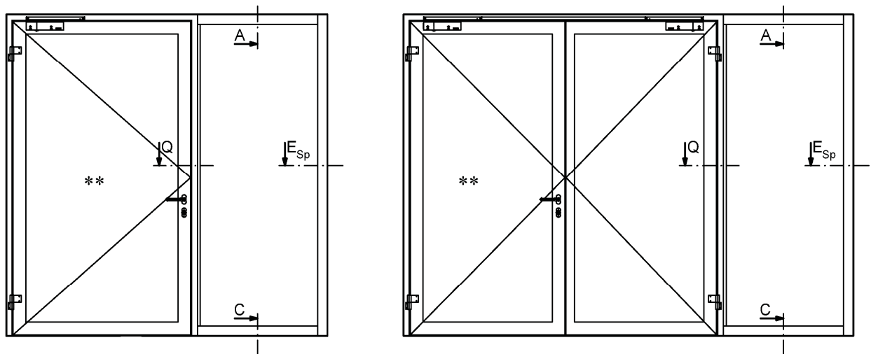
Variante seitlicher Anschluss eines Feuerschutzabschlusses
