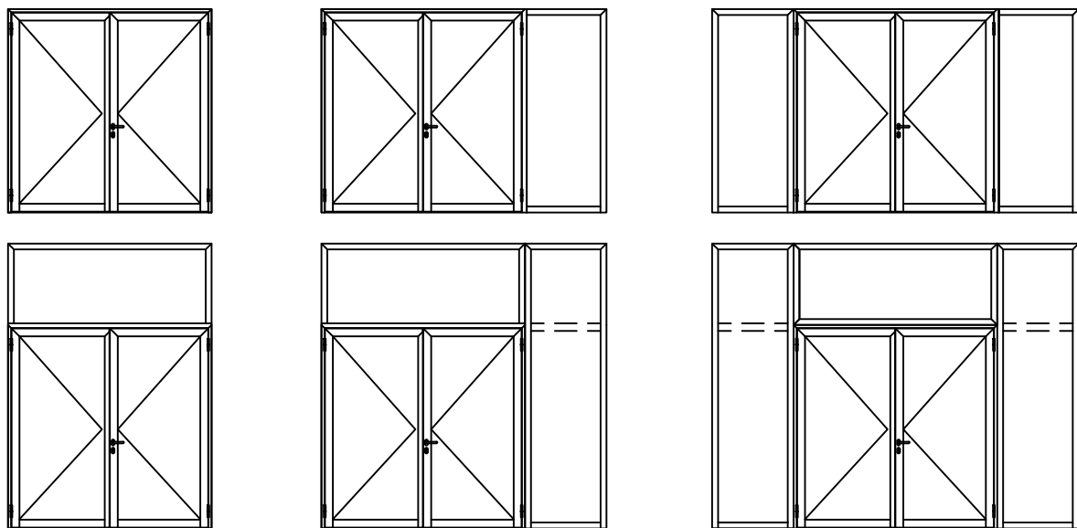
1- flügelig mit Oberlicht und Seitenteil bis 3840 x 4160 (B x H) 2- flügelig mit Oberlicht und Seitenteil bis 5280 x 4160 (B x H)
