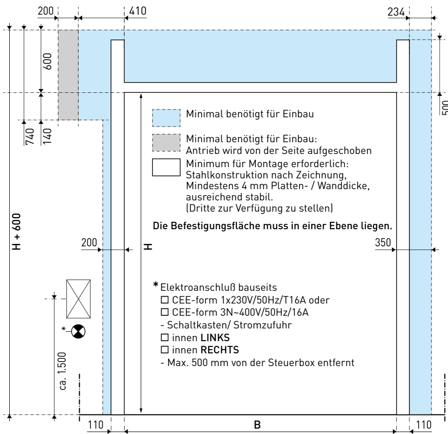
[ Antriebsseite ]
