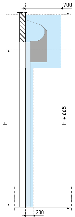
[ Leiterquerschnitt ]
